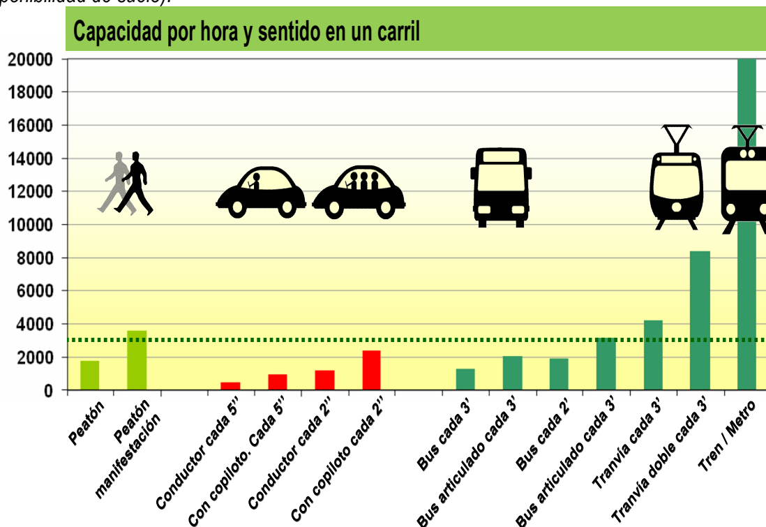
Figura 41. Capacidad de los modos de transporte en zona urbana (el ámbito con menor disponibilidad de suelo).
