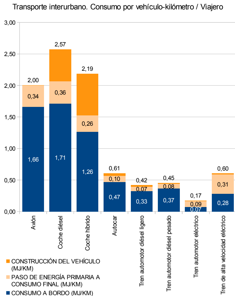
FIGURA A20. Consumo y emisiones por viajero-kilómetro en zona interurbana.
