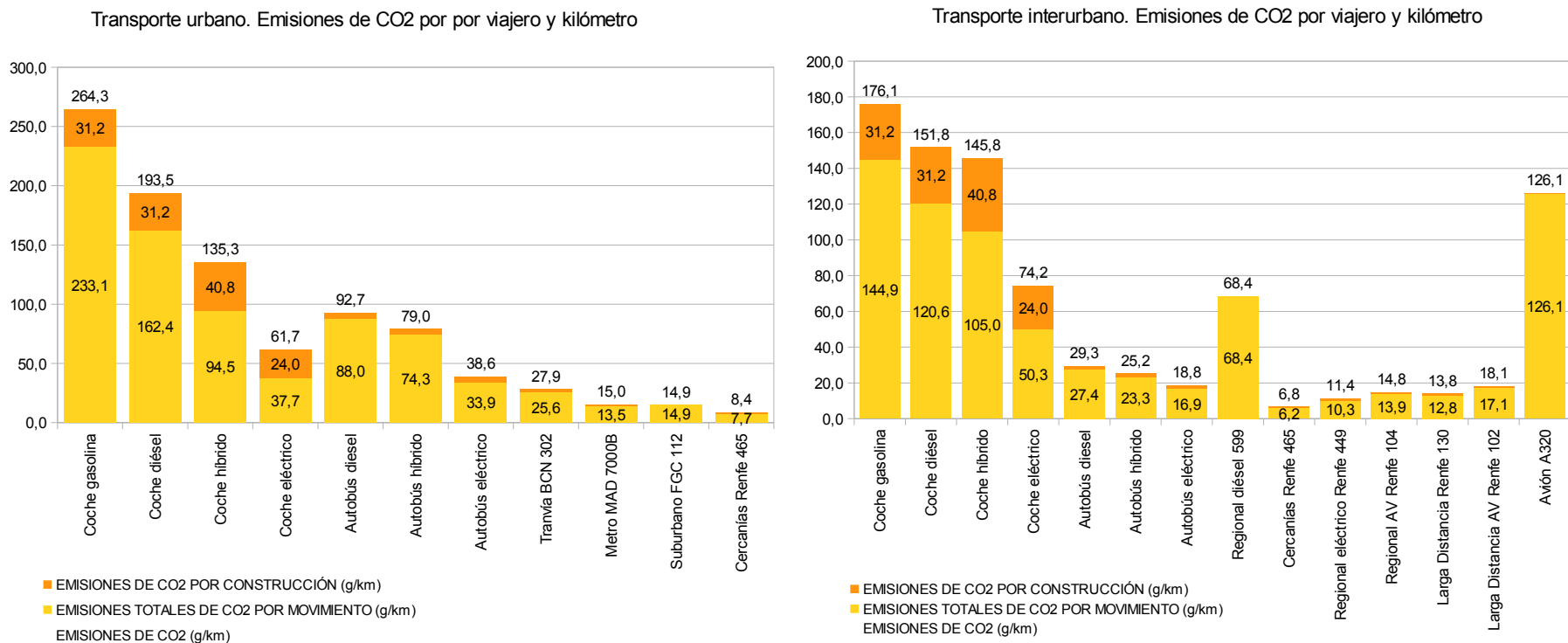
FIGURAS 26 y 27. Emisiones de CO 2 por viajero-kilómetro en zona urbana e interurbana teniendo en cuenta movimiento y construcción de los vehículos.
