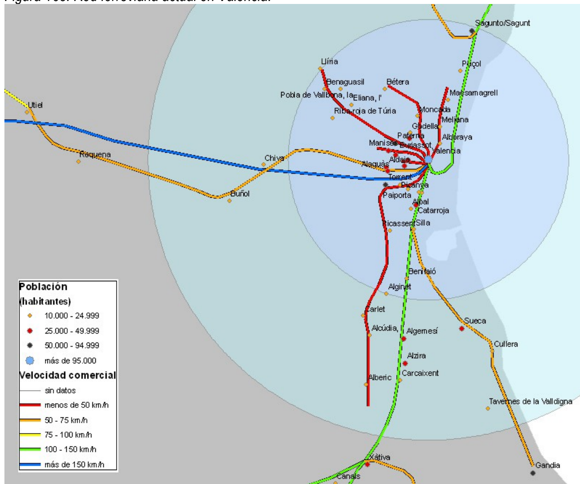
Figura 168. Red ferroviaria actual en València.
