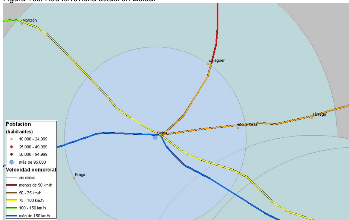
Figura 188. Red ferroviaria actual en Lleida.
