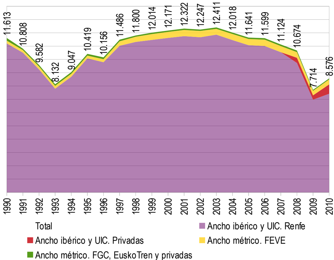
Evolución del tráfico de Renfe, FEVE y operadores autonómicos y privados. Figura 67. Evolución del tráfico de Renfe, FEVE, operadores autonómicos y privados. Expresado en millones de toneladas-kilómetro.
