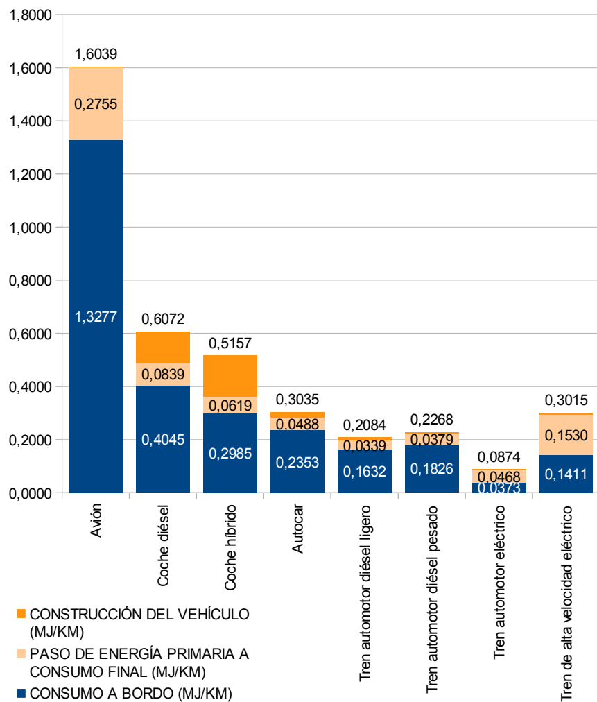
FIGURA A16. Consumo y emisiones por vehículo-kilómetro entre plazas totales en zona interurbana.
