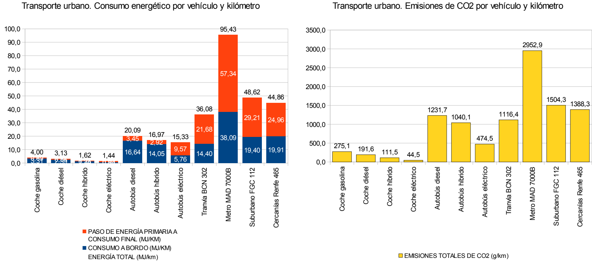
FIGURA A24. Consumo y emisiones por vehículo-kilómetro en zona urbana.
