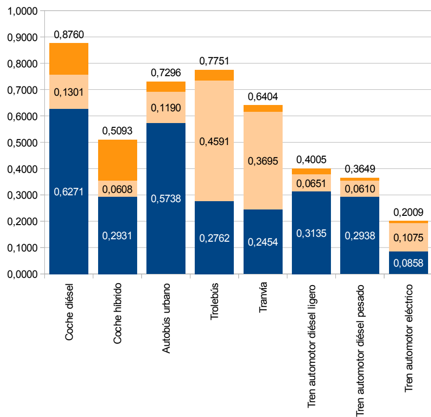
FIGURA A17. Consumo y emisiones por vehículo-kilómetro entre asientos totales en zona urbana.
