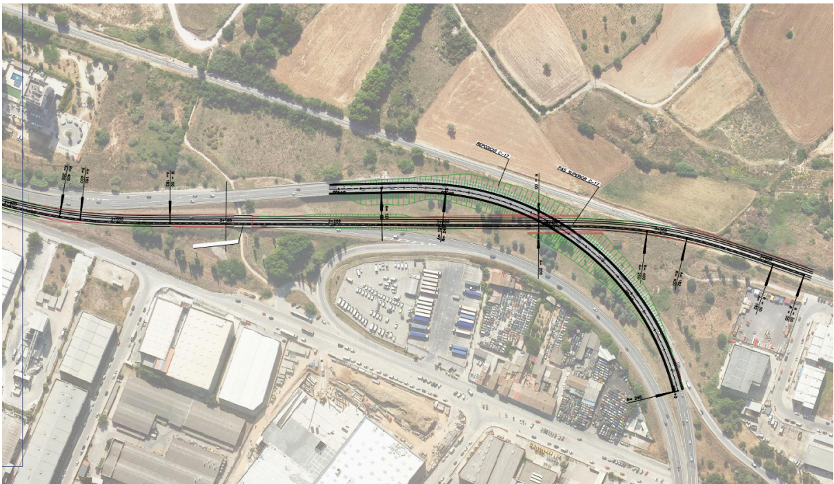
Fig 9: Traçat en planta entre els P.K. 2+900 i 3+600.
